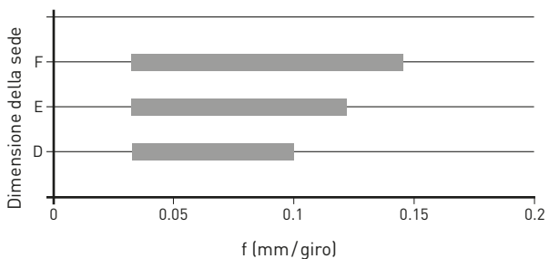
Rompitruciolo R/L05-GM
