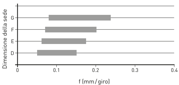
Rompitruciolo R/L05-GM
