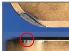
Scheggiatura dopo una lavorazione di 360 secondi
