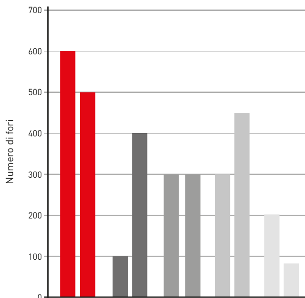
DOPO L'ESECUZIONE DI 300 FORI
