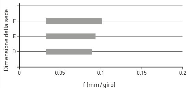
Rompitruciolo R08-GS
